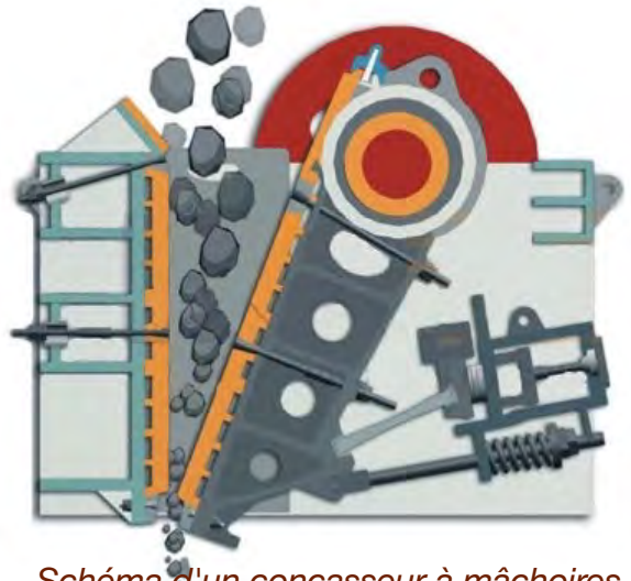
Schéma d'un concasseur à mâchoires
