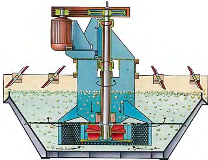
Coupe d'une cellule de flottation
