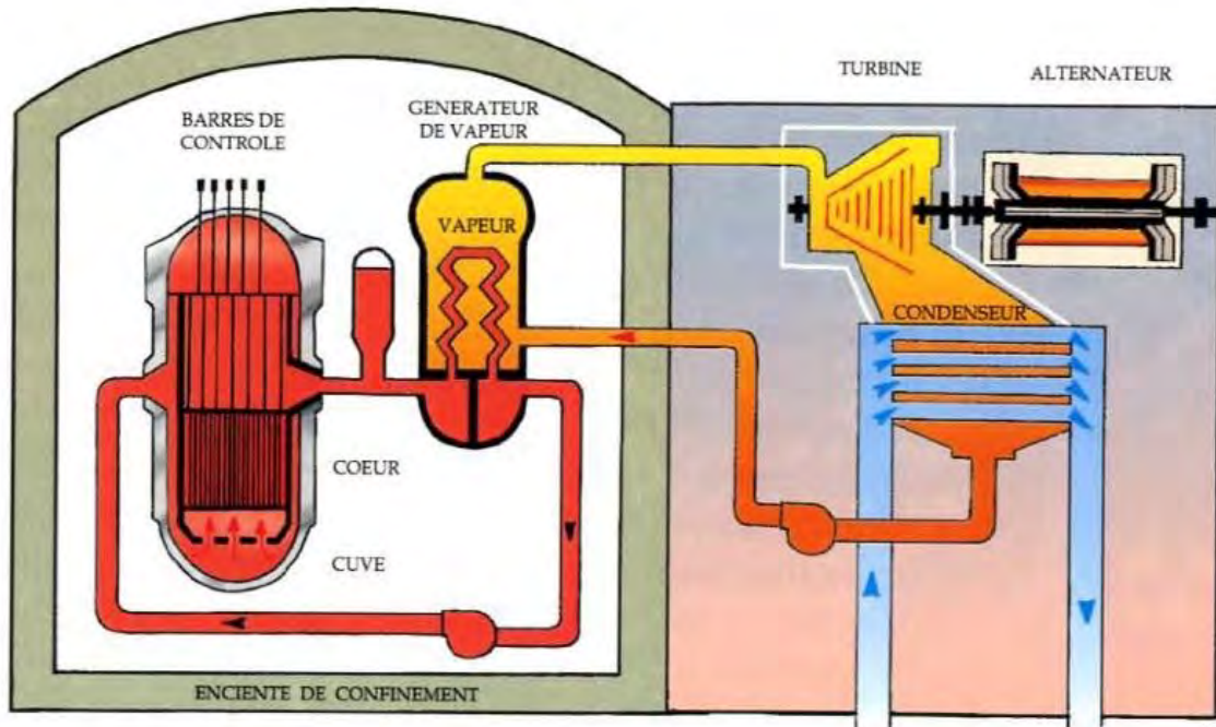
Schéma simplifié du fonctionnement d'une centrale nucléaire
