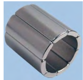
Aimant au néodyme ( Nd_2F_{14}B ) pour rotor de moteur.
