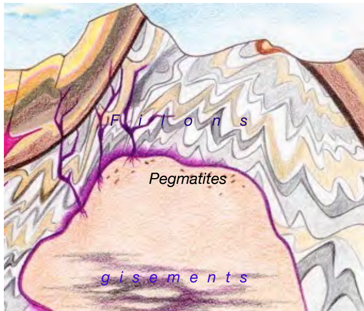
Représentation schématique d'un batholite granitique.
