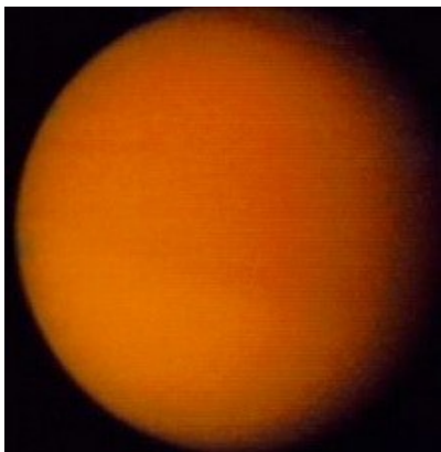
Titan est le plus gros satellite du système solaire.
