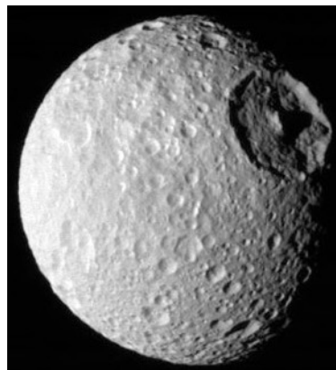
Mimas et son énorme cratère
