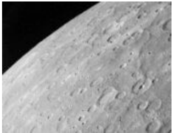
Surface de Mercurure photographiée par la sonde Mariner 10 en 1974
