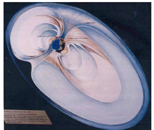
Visualisation du champ magnétique terrestre qui dévie et piège les particules du vent solaire.
