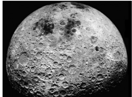
Cratères sur la face cachée de la Lune (photo Apollo 16)
