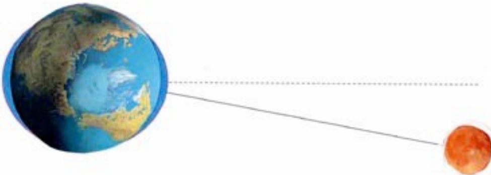
L'ensemble Terre-Lune, un haltère asymétrique. On distingue les deux bourrelets que constituent les marées .
