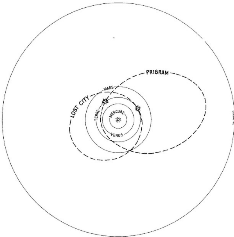
Reconstitution des orbites de deux météorites, Pribram et Lost City. La partie haute de leur orbite se situe dans la ceinture des Astéroïdes.
