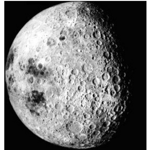
Face cachée de la Lune cartographiée par la sonde Appolo 16 ,en 1972
