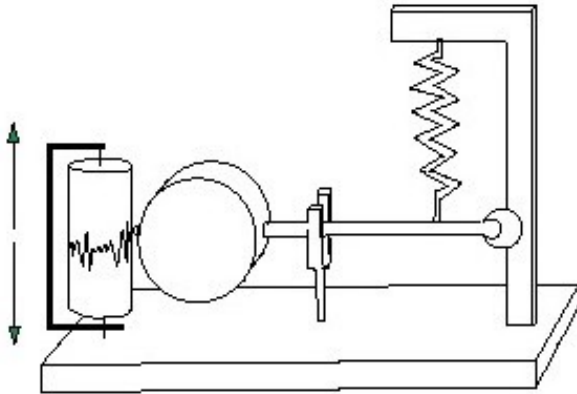
Principe du sismographe mesurant la fréquence et l'amplitude des ondes verticales.
