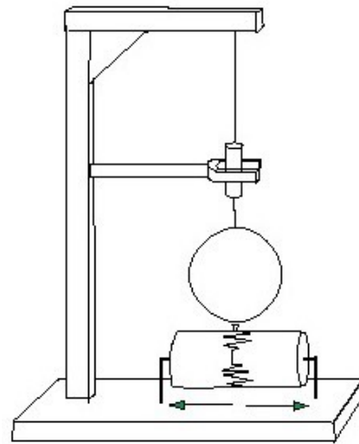
Principe d'un sismographe mesurant la fréquence et l'amplitude des ondes horizontales
