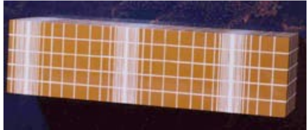
Ondes de compression
