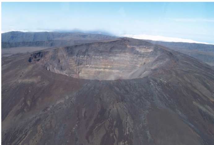
Le Piton de la Fournaise sur l'île de la Réunion est un volcan situé au-dessus d'un point chaud.
