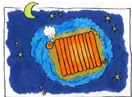
La Terre, un radiateur géant
