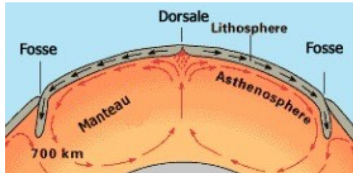
Courants de convections qui expliqueraient le déplacement des plaques lithosphériques
