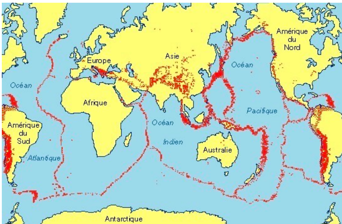
Les principales plaques tectoniques qui morcellent la croûte ter-
