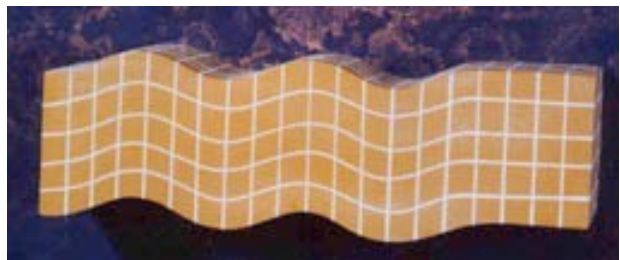
Ondes de cisaillement
